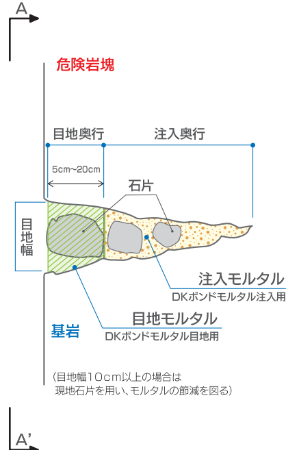
A-A' 施工断面図(亀裂部)
